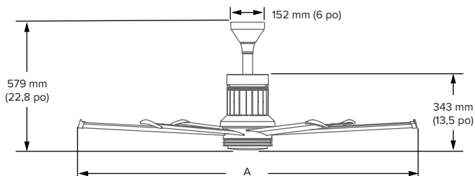
Avec tige de suspension de 152 mm (6 po) et kit d'éclairage 5
