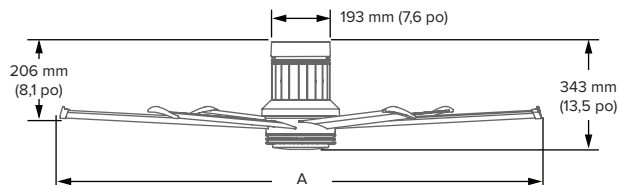
Avec fixation directe et kit d'éclairage 5
