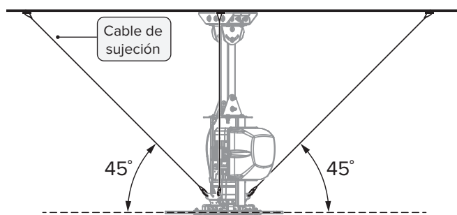
Fig. 2.1: Vista lateral (X-Y)
