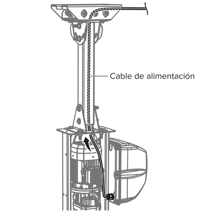
Fig. 3: Tendido del cable de alimentación
