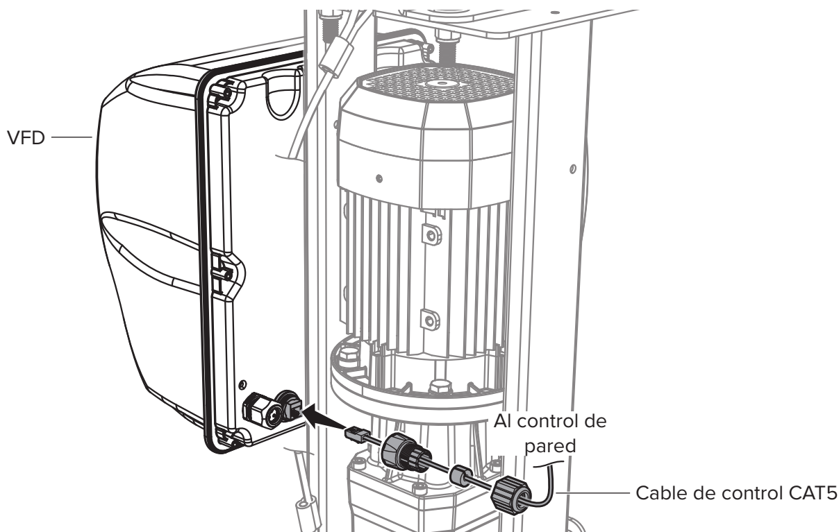
Fig. 1: Cable de control CAT5 al VFD
