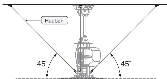
Fig. 2.1 : Vue latérale (X-Y)
