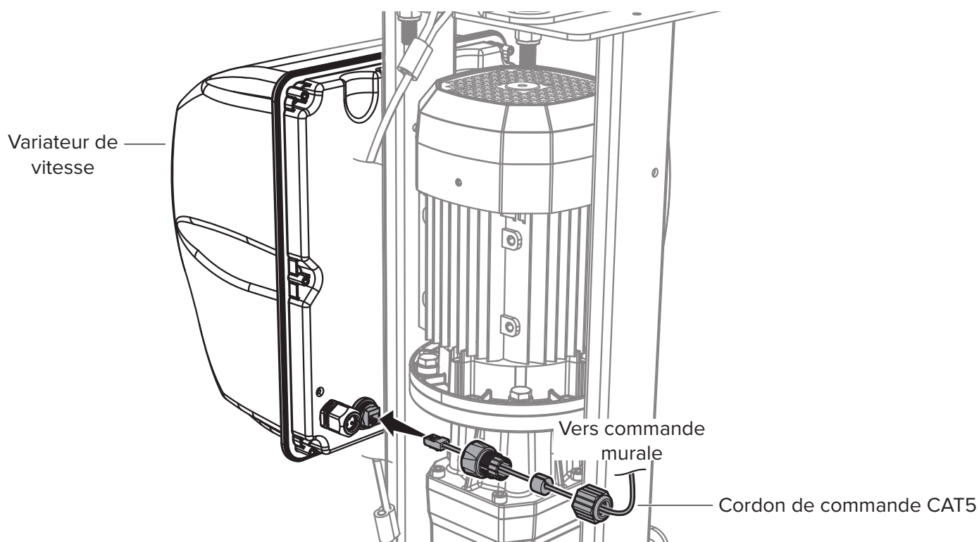
Fig. 1 : Cordon de commande CAT5 vers variateur de vitesse
