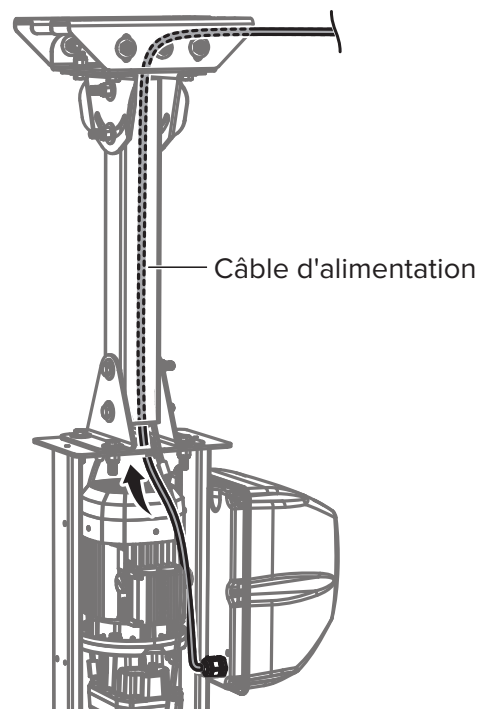
Fig. 3 : Acheminement du câble d'alimentation
