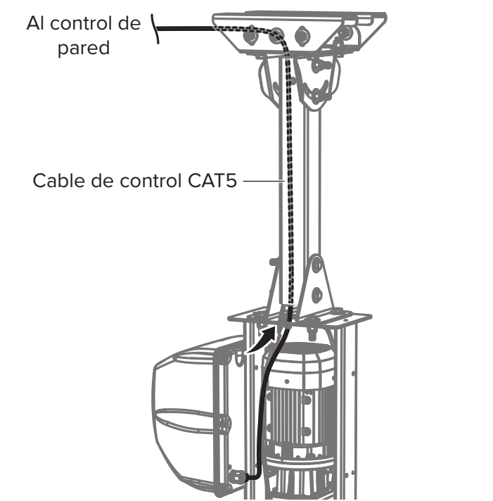
Fig. 2: Tendido del cable de control CAT5
