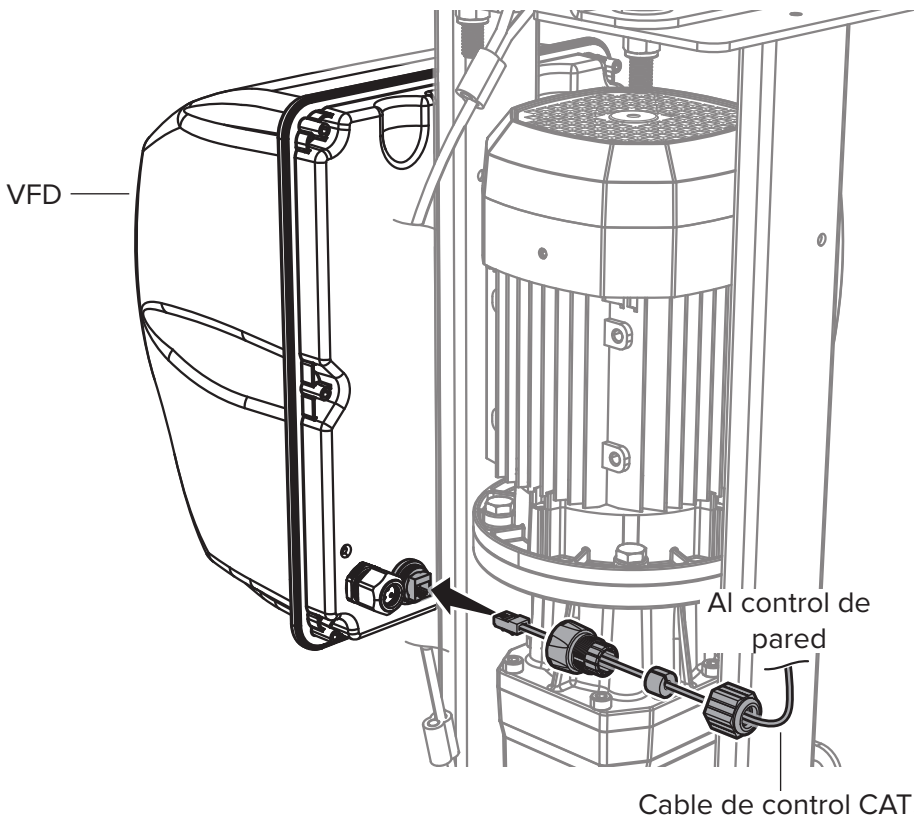
Fig. 1: Cable de control CAT5 al VFD
