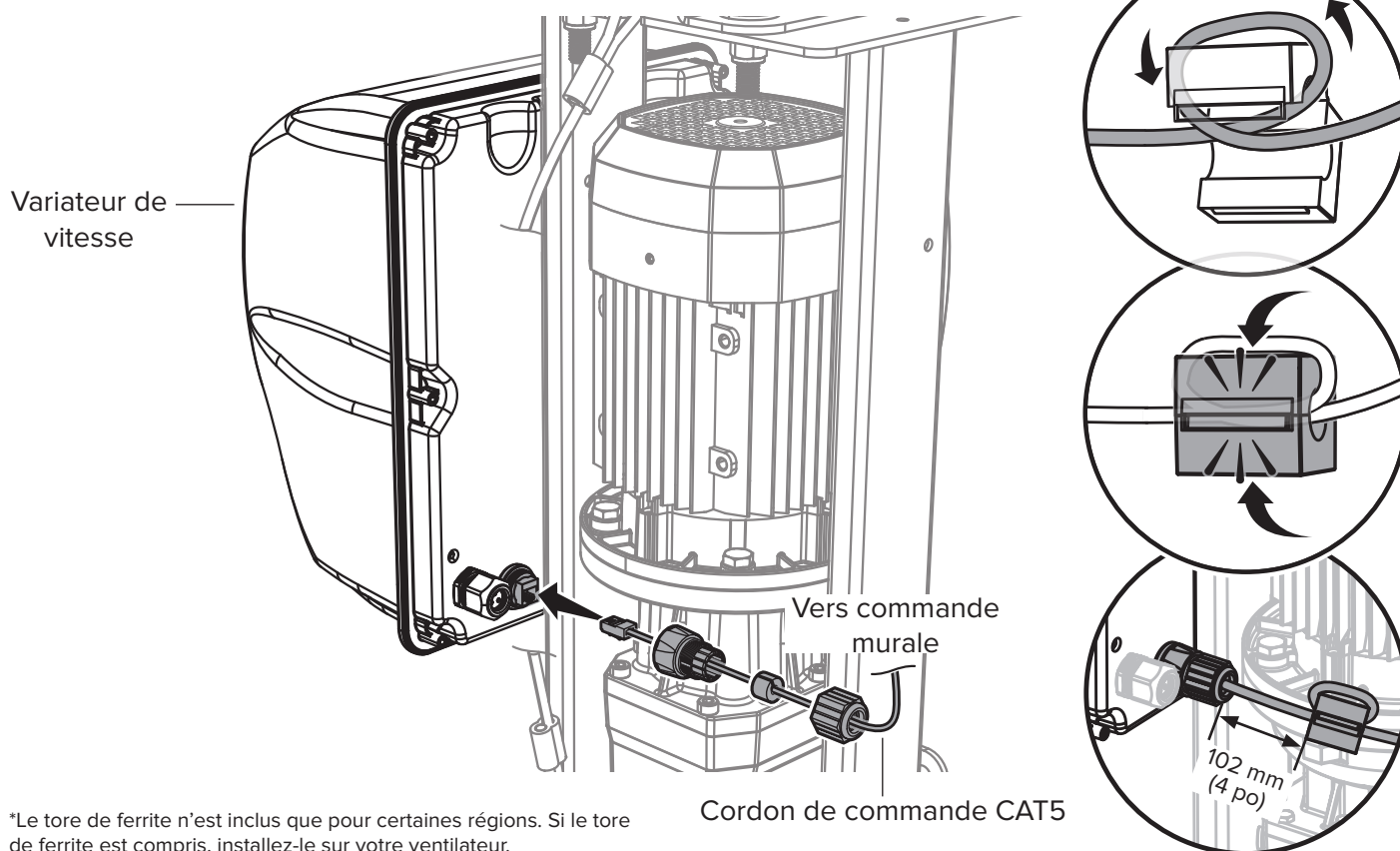
Fig. 1 : Cordon de commande CAT5 vers variateur de vitesse
